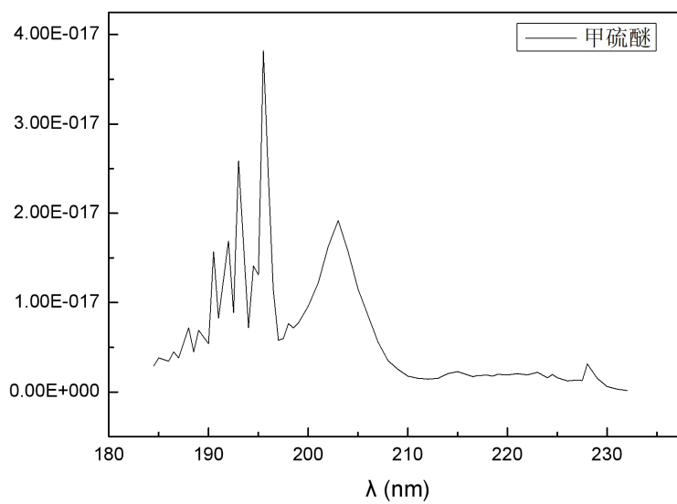
图 C.4 甲硫醚的紫外吸收光谱
