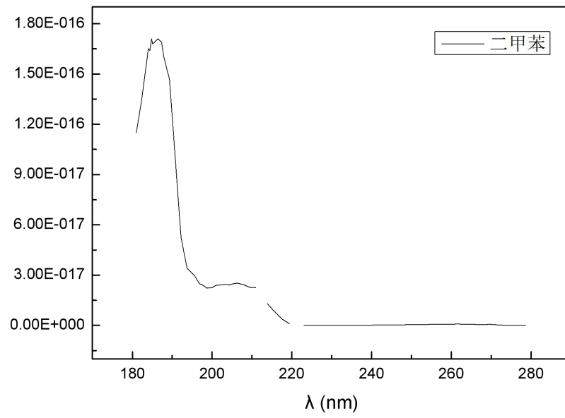
图 C.5 二甲苯的紫外吸收光谱
