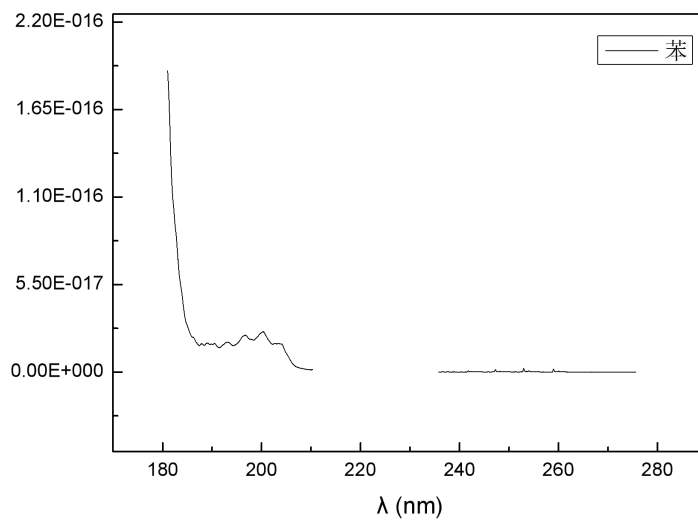
图 C.3 苯的紫外吸收光谱
