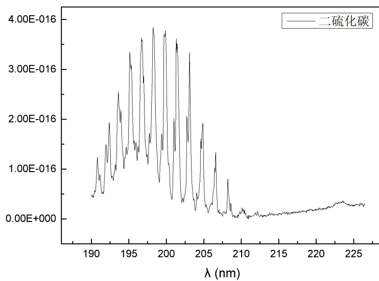
图 C. 12 二硫化碳的紫外吸收光谱
