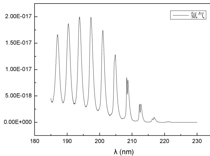
图 C. 2 氨气的紫外吸收光谱
