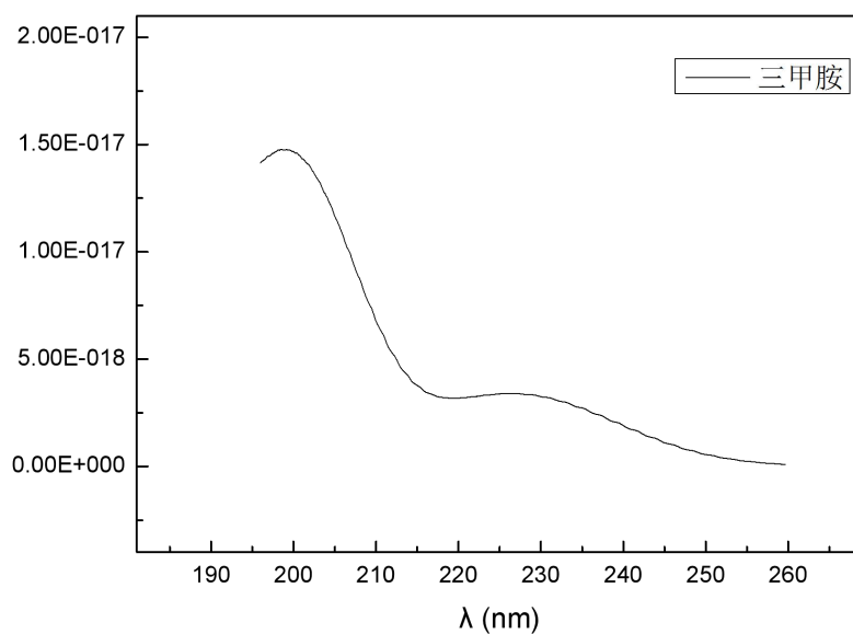
图 C. 11 三甲胺的紫外吸收光谱
