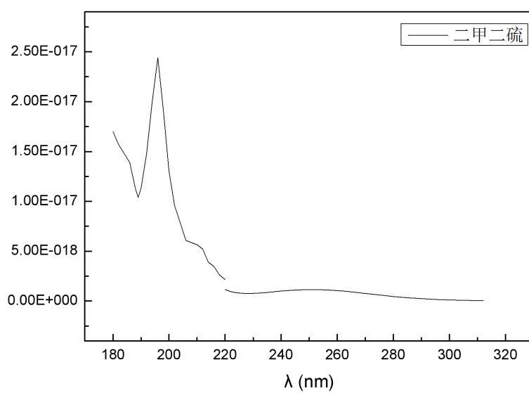
图 C.10 二甲二硫的紫外吸收光谱
